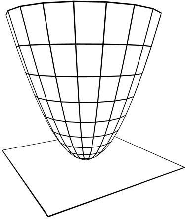
Paraboloïde elliptique (au-dessus de son plan tangent)
