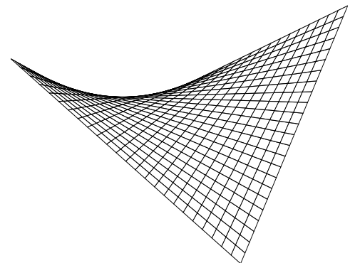
Autre visualisation des droites
