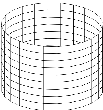
cylindre elliptique
