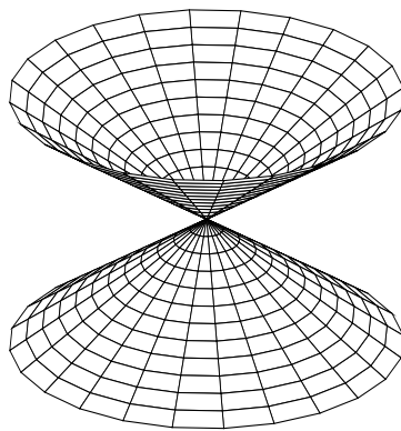
cône du second ordre
