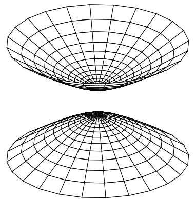
hyperboloïde à deux nappes
