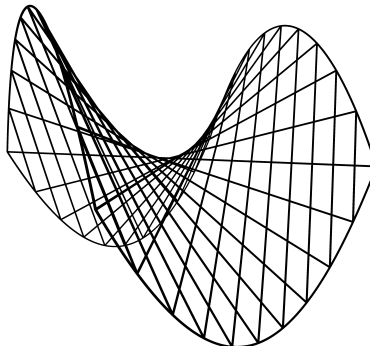
Visualisation des droites
