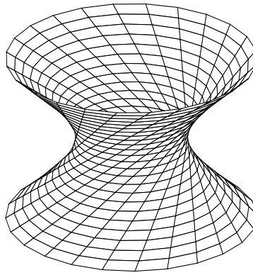
Première famille de droites
