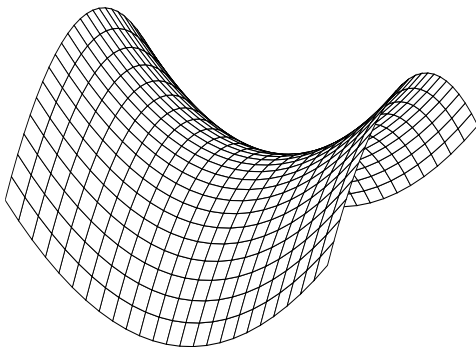
Paraboloïde hyperbolique
