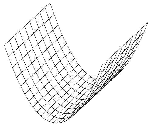
cylindre parabolique
