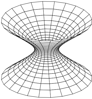
Hyperboloïde à une nappe
