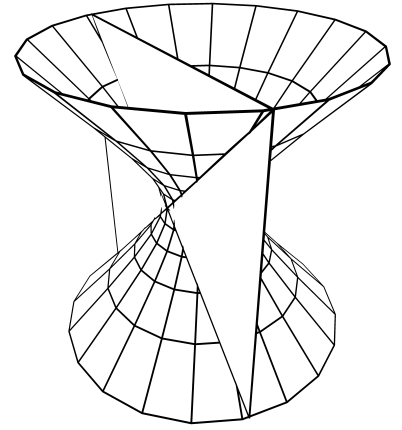
Hyperboloïde à une nappe (traverse son plan tangent)
