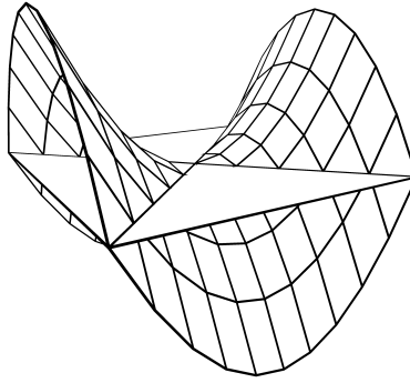
Paraboloïde hyperbolique (traverse son plan tangent)
