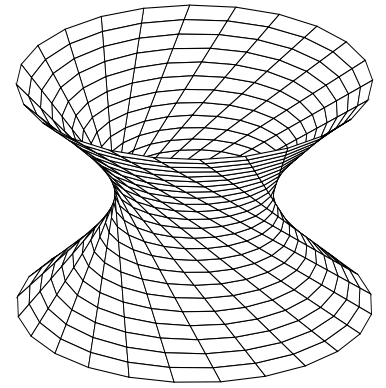
Deuxième famille de droites
