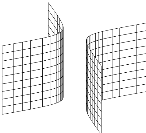
cylindre hyperbolique
